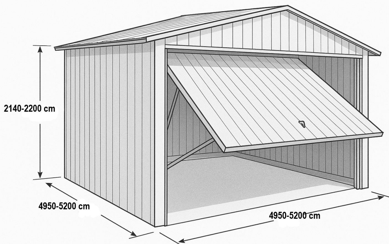
GARAŻ BLASZANY Z DACHEM DWUSPADOWYM
